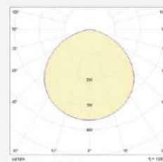
AC1411 Óptica 110°
