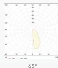
FOTOMETRÍA
